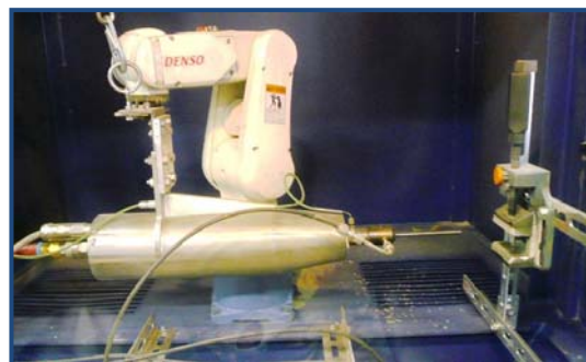
スプレーブース内 ACGS ガンヘッド
